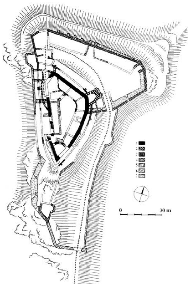
Čachtický hrad – pôdorys s vyznačením stavebného vývoja: 1 – jadro z 13. storočia, 2 až 4 – 14. až prvá polovica 15. storočia, 5 – druhá polovica 15. storočia, 6 a 7 – 16. a 17. storočie
